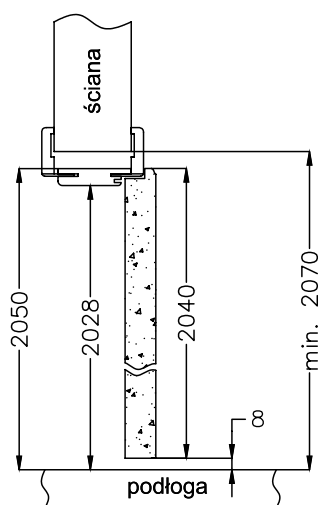
Przekrój OR z kątownikiem 60
